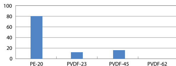
图2 不同品种和膜厚彩涂钢板 QUUV 试验 3000 小时后失光率对比
