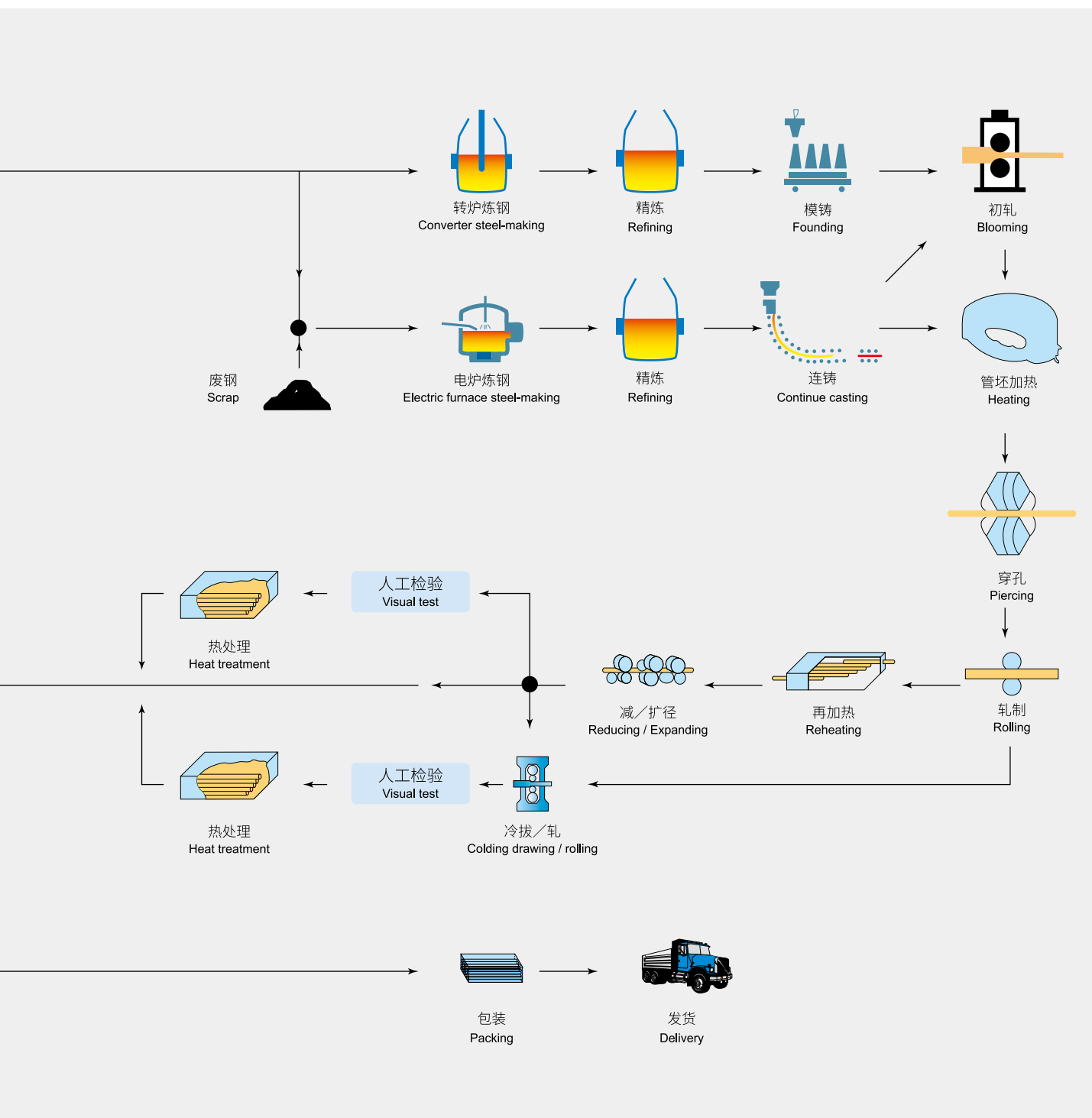
无缝管线管工艺流程图
