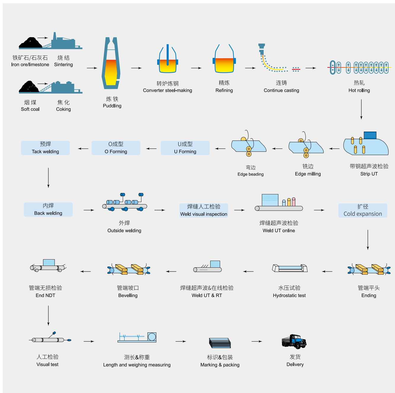
UOE 管线管工艺流程图
