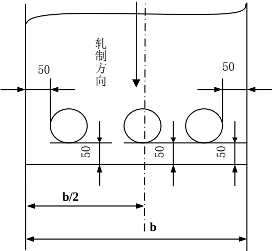
图 1 镀层重量试样的取样位置，b 为钢板或钢带的宽度，单位为 mm。
