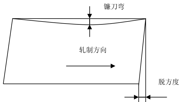
图 A.1 脱方度和镰刀弯
